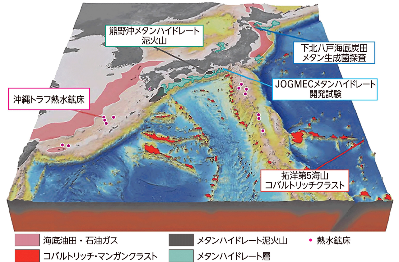
[出所:浦辺徹郎ほか原図(2012)]
